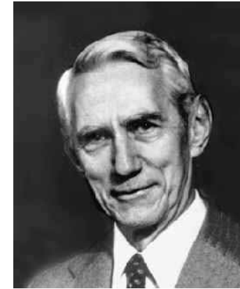
Shannon (1916-2001)
